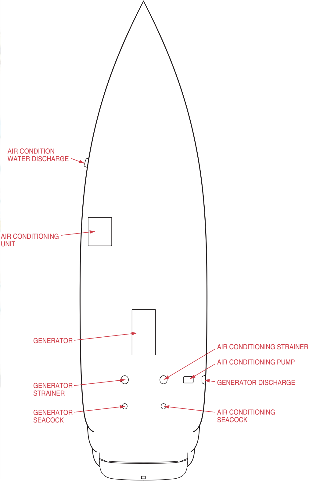
COB_0121_A
