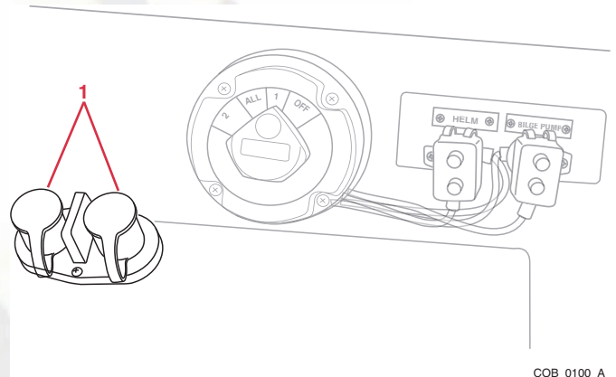
1 – Receptacle
