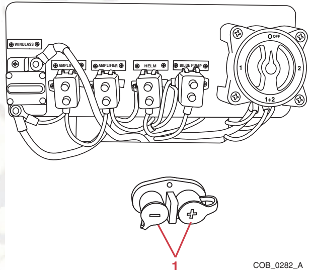
1 – Receptacle
